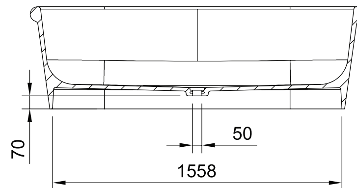
A-A (1:20)
