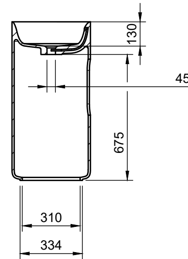
A-A (1:20)
