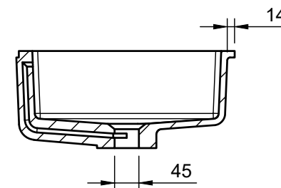
A-A (1:10)
