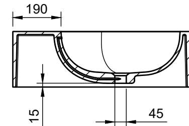
A-A (1:15)
